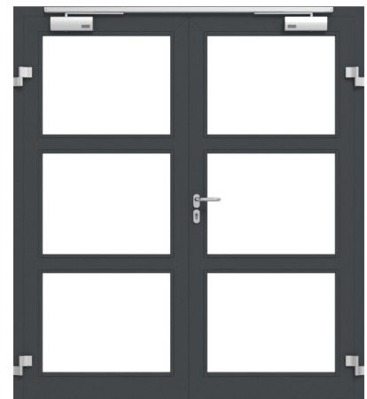
RS 150 LA-03 (2-flg.) mit vier Quersprossen
