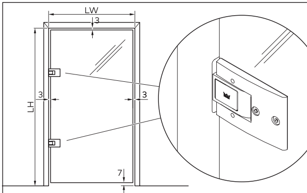
Abb. 8 Spaltmaße für Zargenbefestigung mit eingelassener Montageplatte
