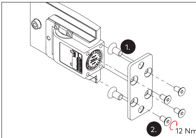
Abb. 24 Befestigung der Montageplatten am Pendeltürband
