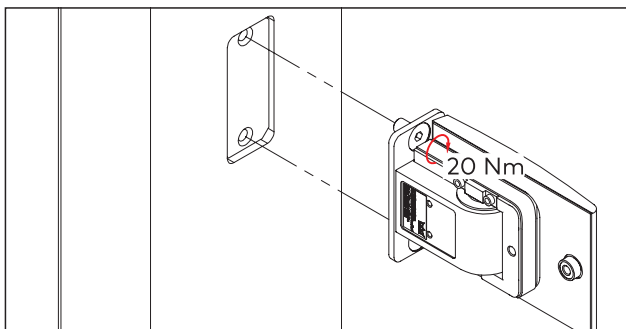
Abb. 25 Montage der Pendeltürbänder in der Zarge
