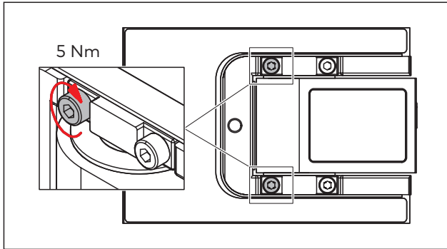
Abb. 15 Die gekennzeichneten Schrauben mit Drehmoment anziehen
