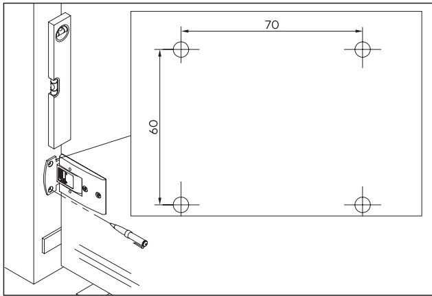
Abb. 19 Bohrbild des Pendeltürbands
