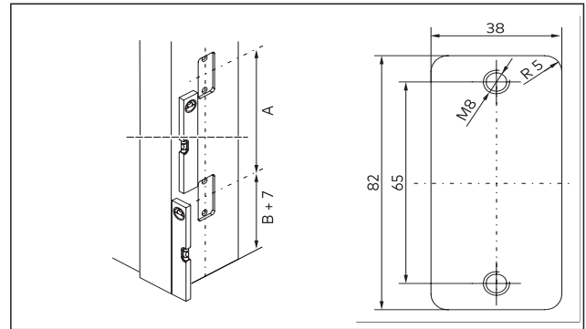
Abb. 21 Maßbild für Aussparungen der Montageplatten in der Zarge
