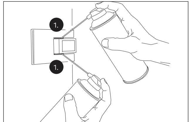
Abb. 37 Schmierung der Laufbuchsen am Drehpunkt
