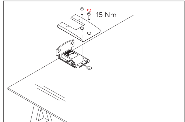
Abb. 17 Befestigung des Pendeltürbands am Glastürflügel
