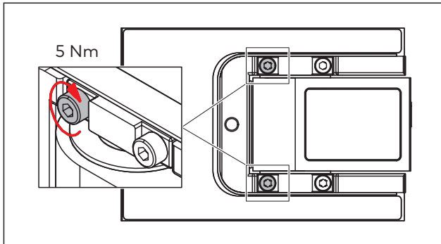
Abb. 23 Die gekennzeichneten Schrauben mit Drehmoment anziehen
