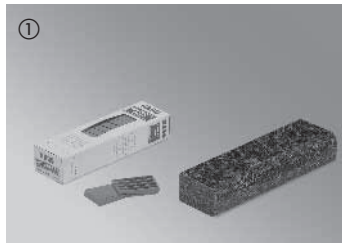
Verlegewerkzeug: Schlagklotz, Abstandskeile, Bleistift, Säge.
