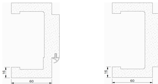
Querschnitt Montagezarge EE
