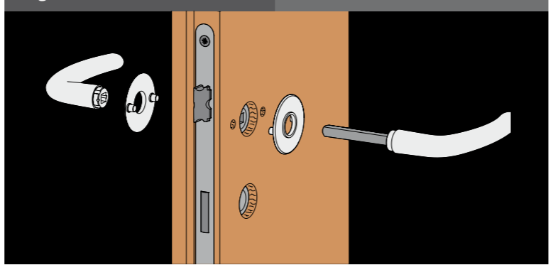
Türgriffe zusammenstecken
